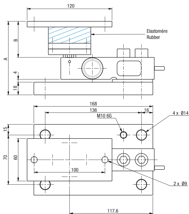
Encombrement et fixation - Dimensions and fixing
