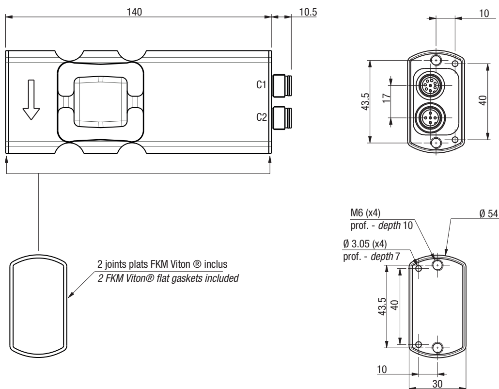
connecteurs 5 poles
