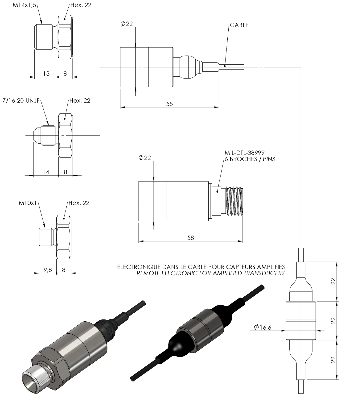
Dimensions : mm
