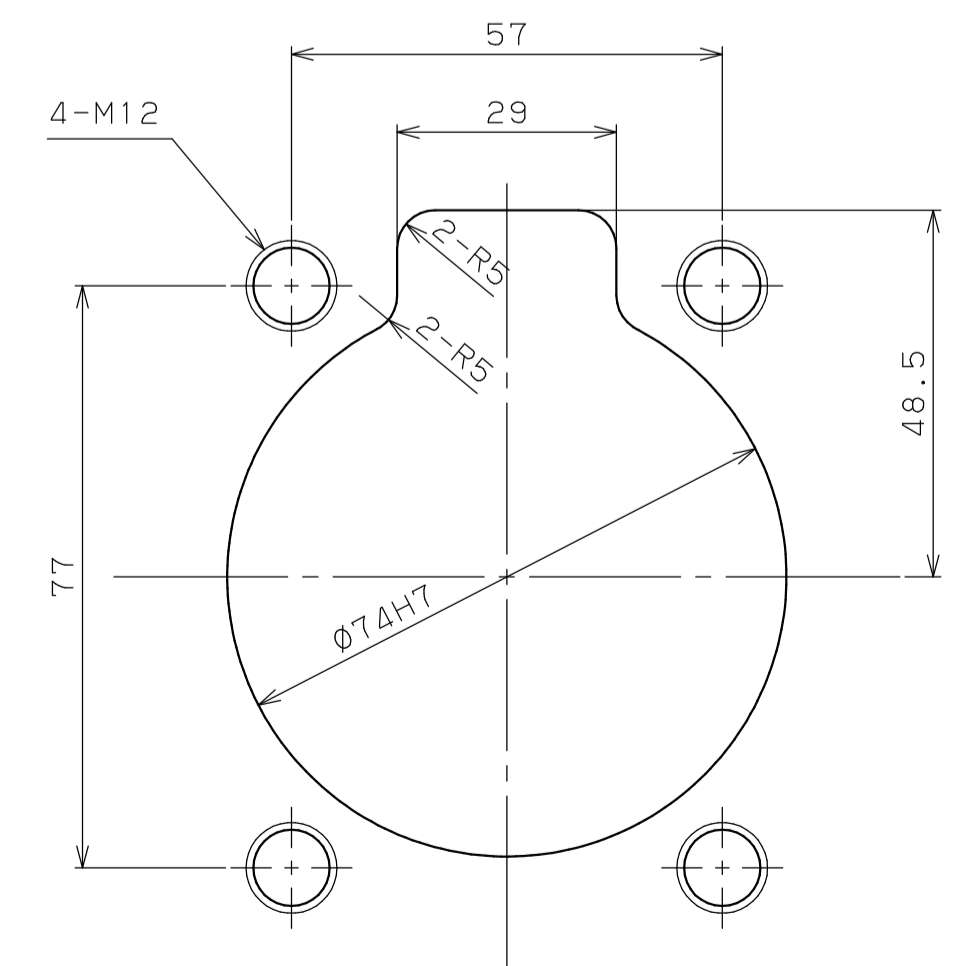
CS20 推奨取付寸法 (2倍図)
